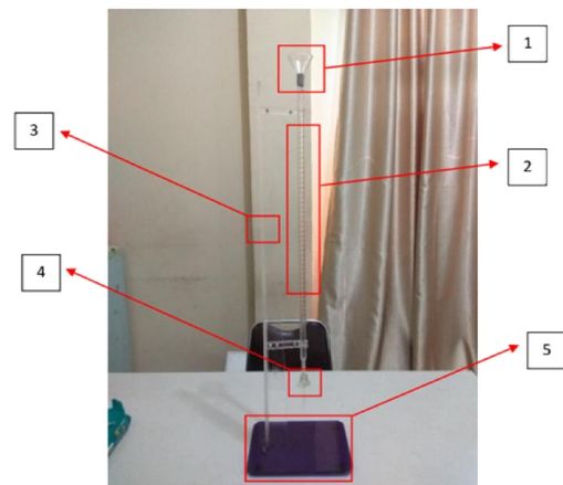
Gambar 2. Hasil rancangan viskometer ostwald alternatif.
