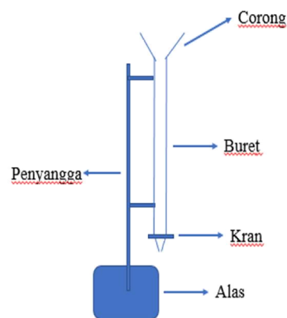
Gambar 1. Desain alat viskometer Ostwald alternatif.
